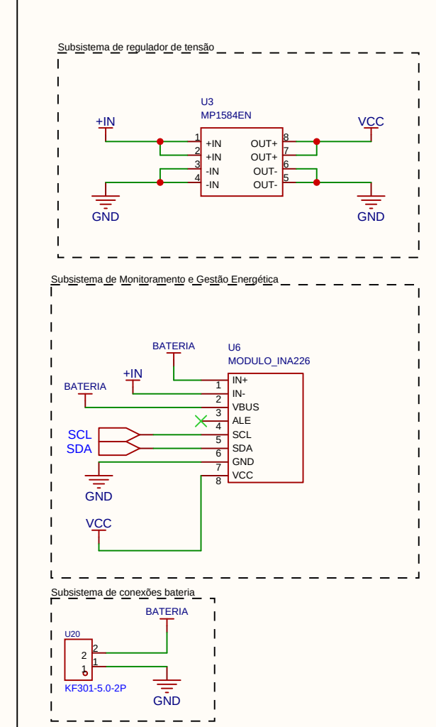
Sistema de energia
