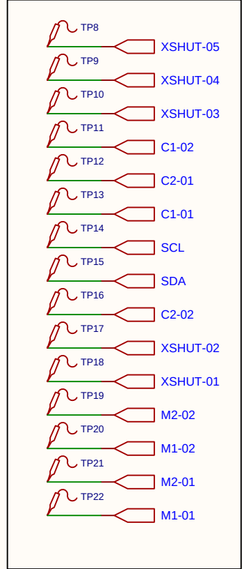
Conexões Test point
