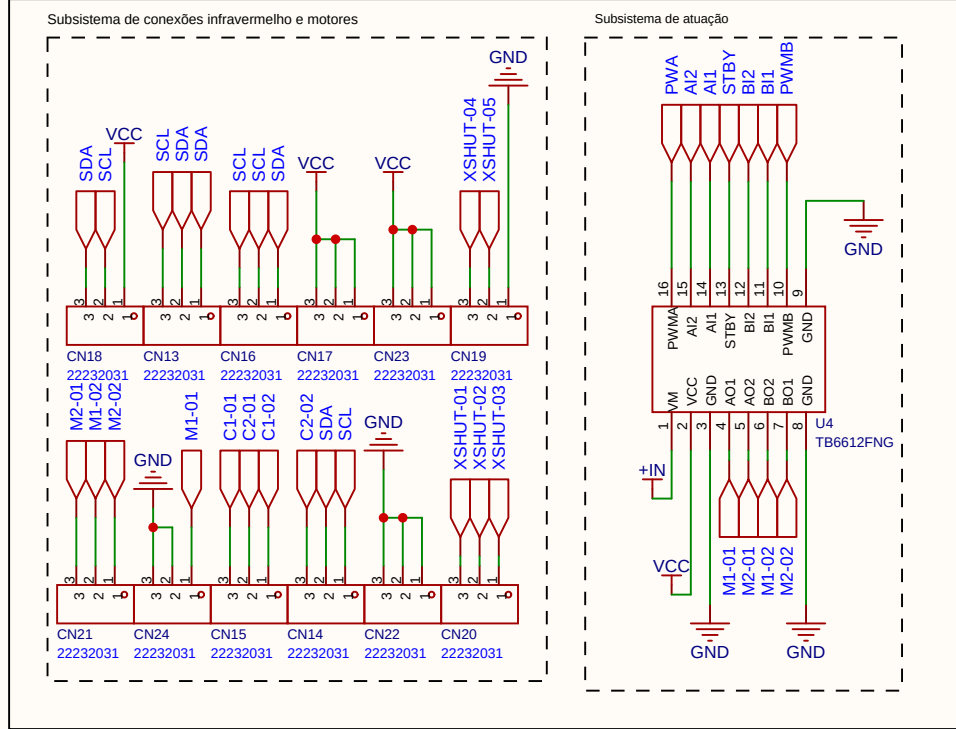
Sistema de sensores de Navegação e de Atuação e Odometria
